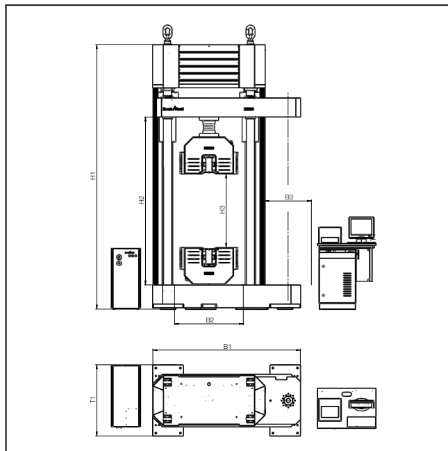
Zeichnung: Z2000ES mit Hydraulik-Probenhalter
