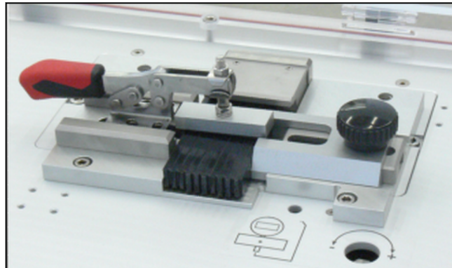
Auswechselbares Probenmagazin
